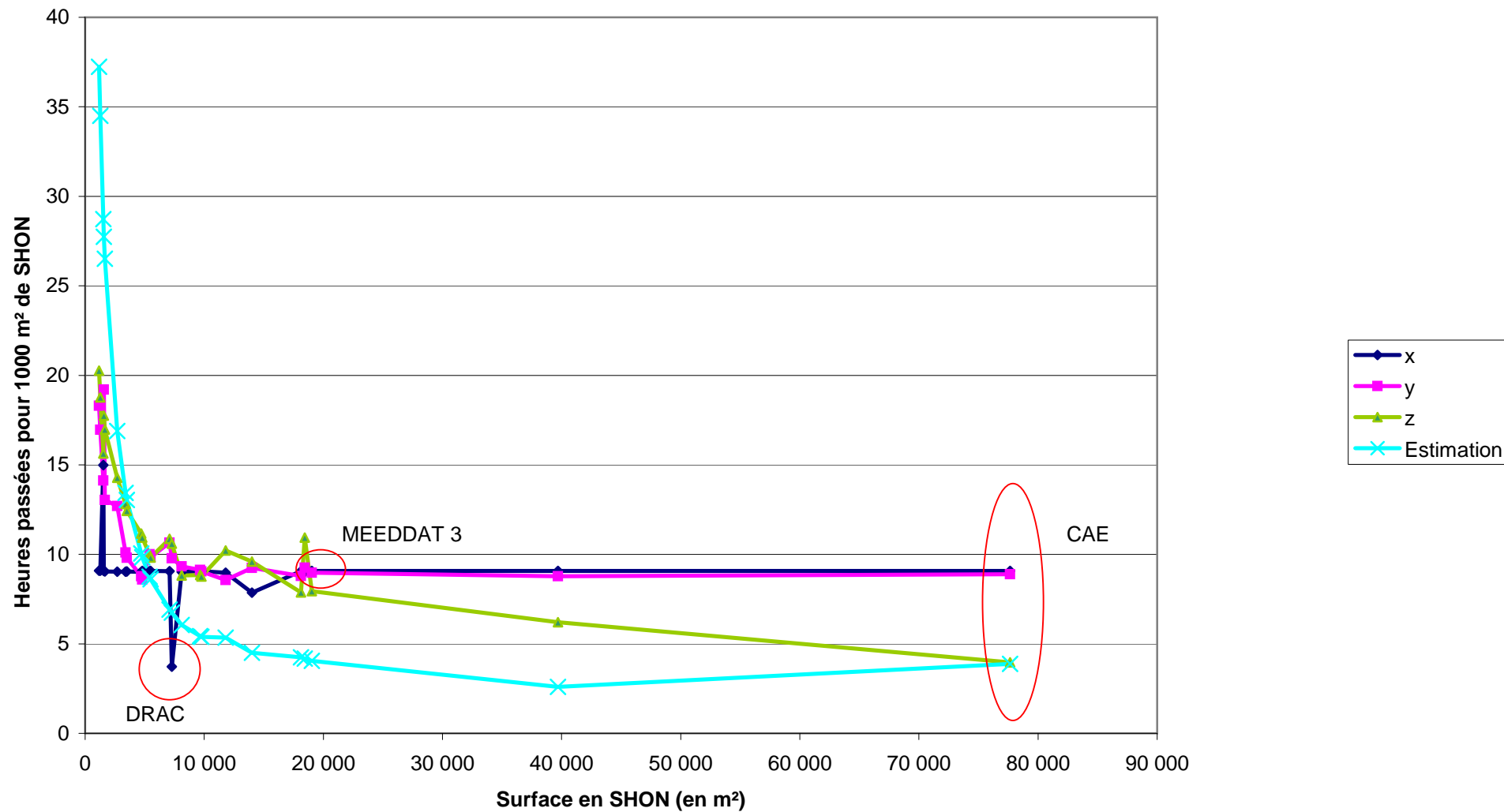
Evolution du temps passés (heures/1000m 2 ) en fonction de la surface du bâtiment
